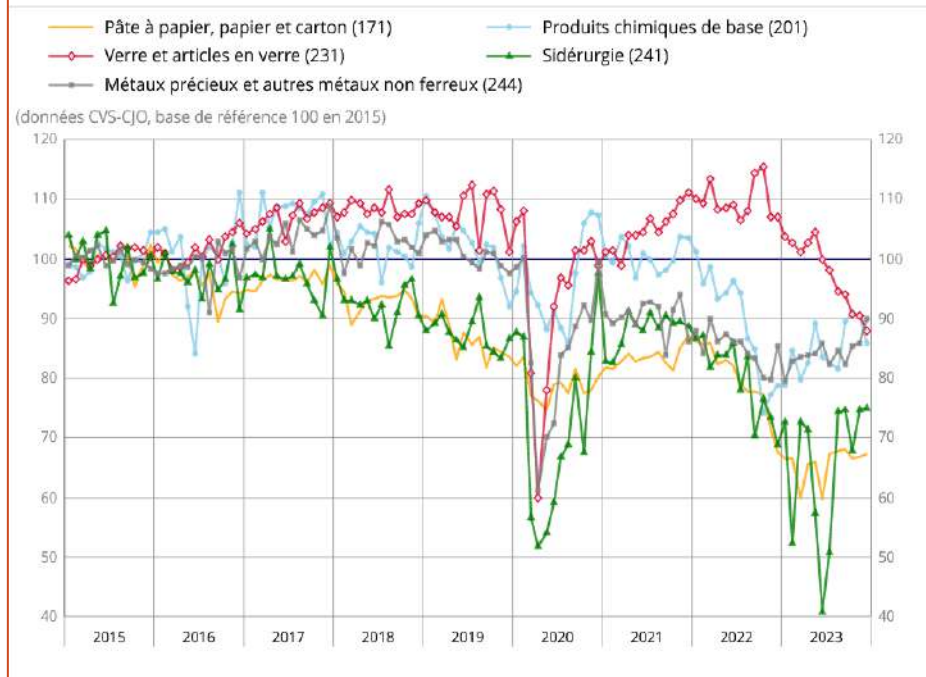
Indices mensuels de production industrielle dans 5 branches intensives en énergie (base 100 en 2015)
