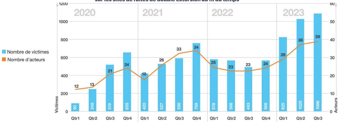
Cyber-extorsion dans le temps : nombre de victimes et d'acteurs observés sur les sites de fuites de double extorsion au fil du temps
