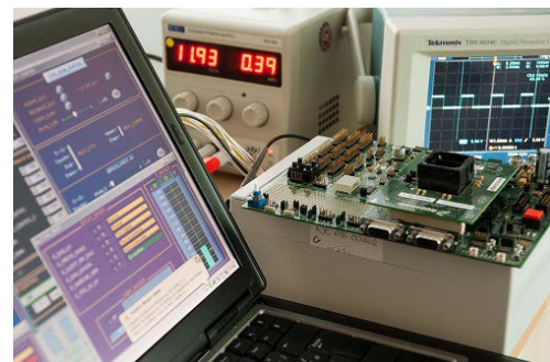
Performances et sûreté de fonctionnement des systèmes embarqués temps-réels avec la méthode de conception PharOS : démonstration sur un ordinateur habitacle embarqué automobile bi-cœur © Philippe Stroppa / CEA (StudioPons)
